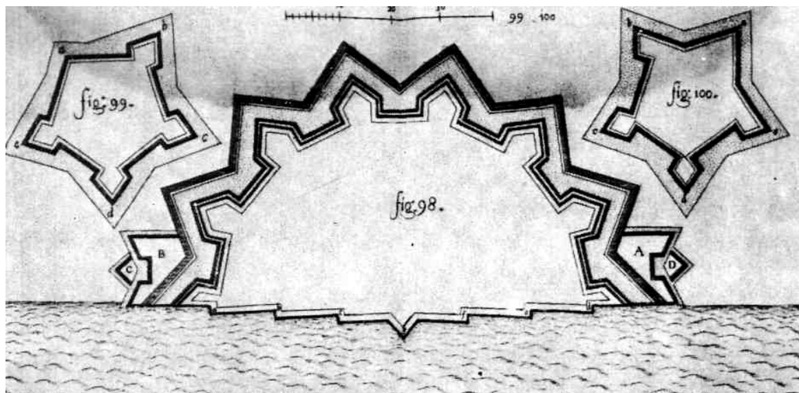
Мал. 6. Адам Фрэйтаг. Умацаванне горада, змешчанага над ракой значнай шырыні 2
