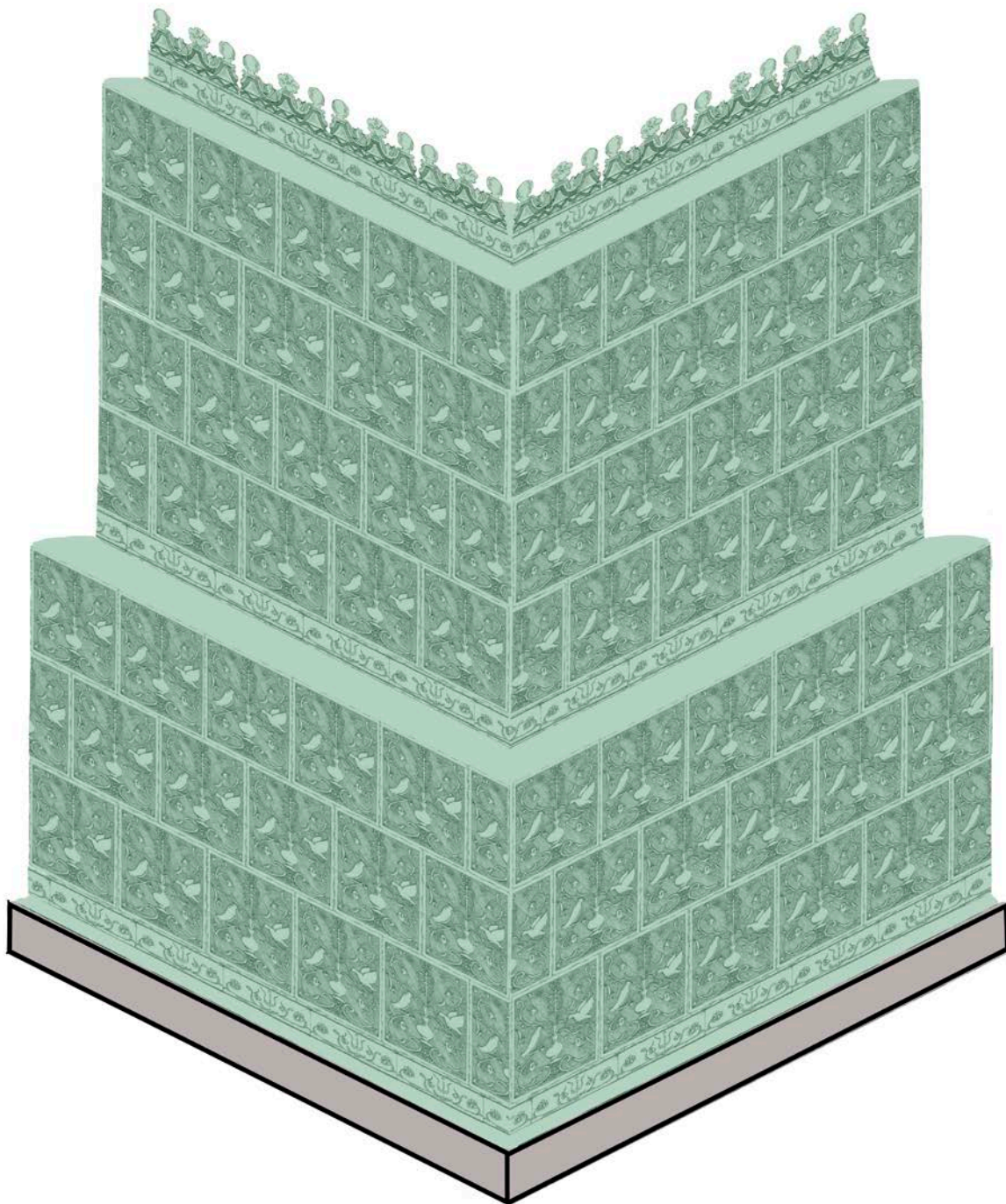
Мал. 39. Ізамерыя кафлянай печы XVII ст. замка ў Старым Быхаве (зялёнай заліўкай без малюнка пазначаны элементы пячнага набору, якія сёння не знойдзены) (рэканструкцыя Н. П. Шутковай)
