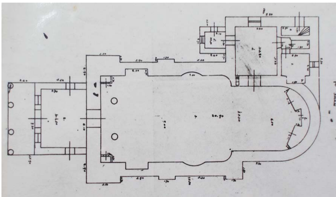
Мал. 22. План касцёла ордэна кармелітаў 1756–1761 гг. у Быхаве 1
